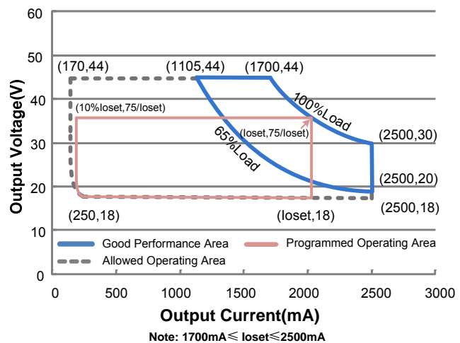
EBD-075S250DV
