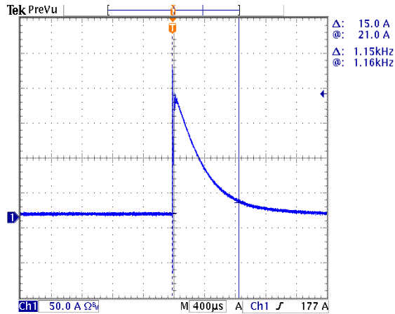
ESD-600S170DT (Io=1360mA)
