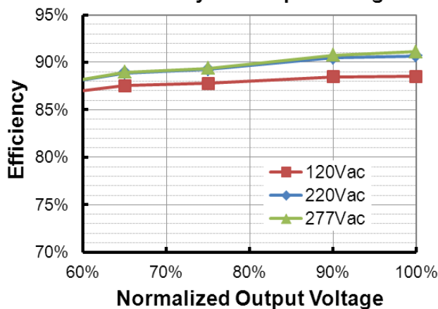
EUD-075S175BT (Io=1190mA)
