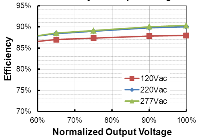
EUD-075S175BT (Io=1750mA)
