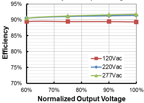
HUK-096S210DV( I_o=1400mA )
