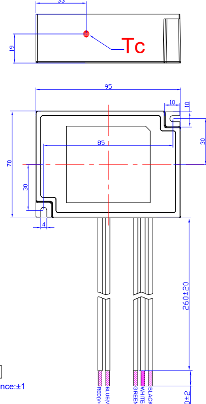
LUN-042SxxxST
