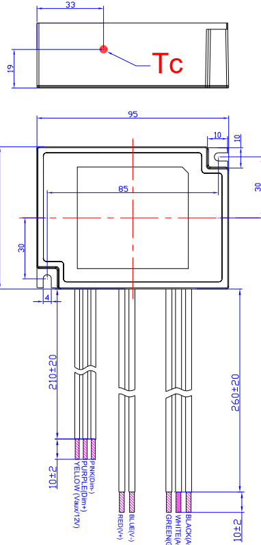
LUN-042SxxxDT
