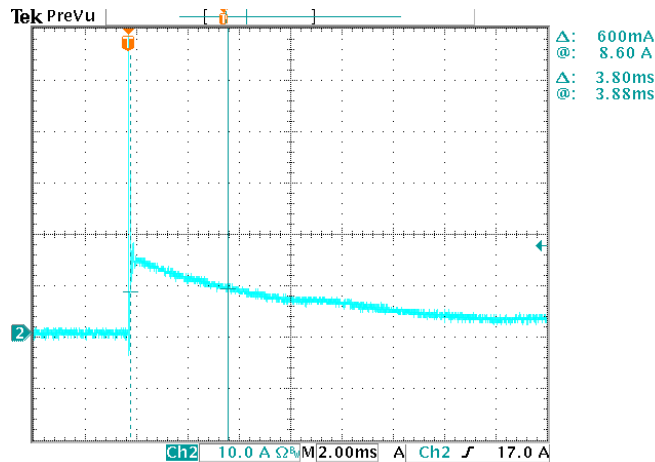
SUM-1K5S12AMx(Io=10000mA)
