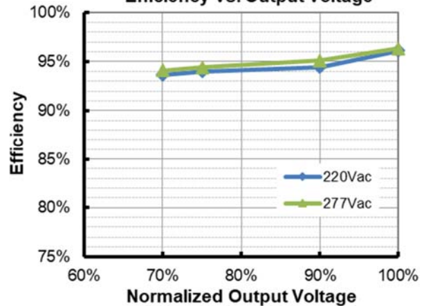
SUM-1K5S31AMx(Io=31500mA)
