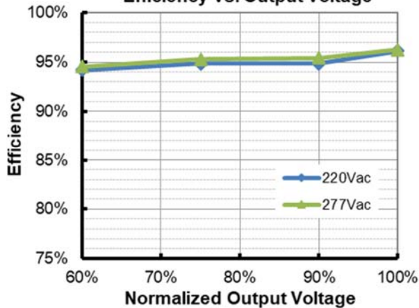
SUM-1K5S31AMx(Io=28000mA)
